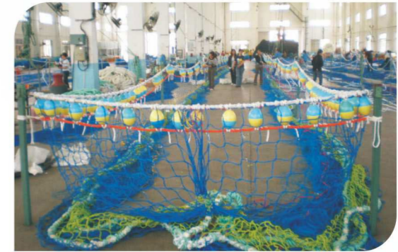
Danish Seine net Assembling 三腳虎網組合成品
