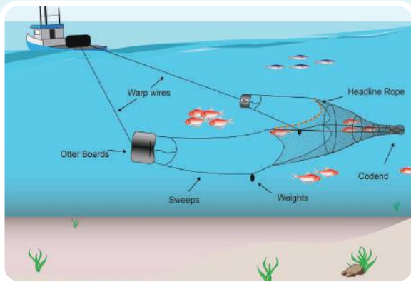
Trawl Net / 拖網
